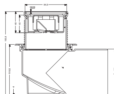
Ø 100 HORIZONTAL OUTLET
