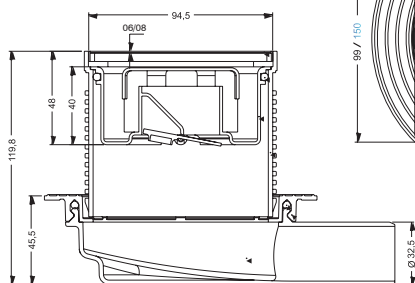
Ø 32 HORIZONTAL OUTLET
