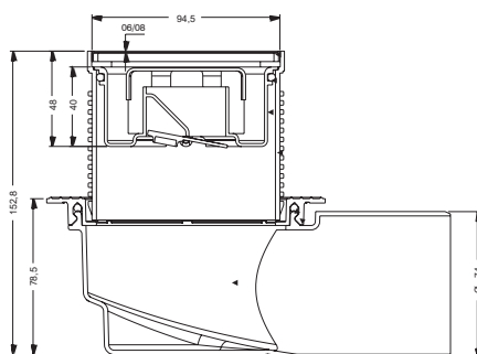
Ø 70 HORIZONTAL OUTLET
